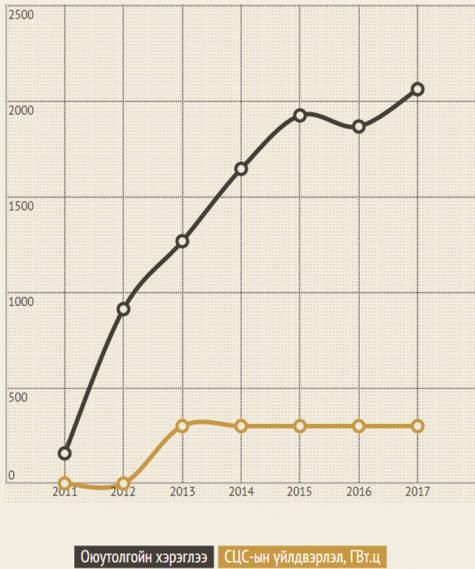
График-4. Салхин цахилгаан станцын үйлдвэрлэлийг Оюутолгойн хэрэглээтэй харьцуулсан байдал
